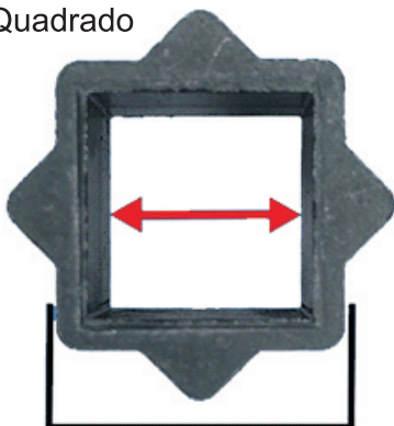
2ª Medida Diâmetro Externo do Quadrado
